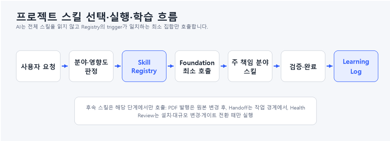
그림 1. 요청부터 Learning Log까지의 선택적 호출 흐름
